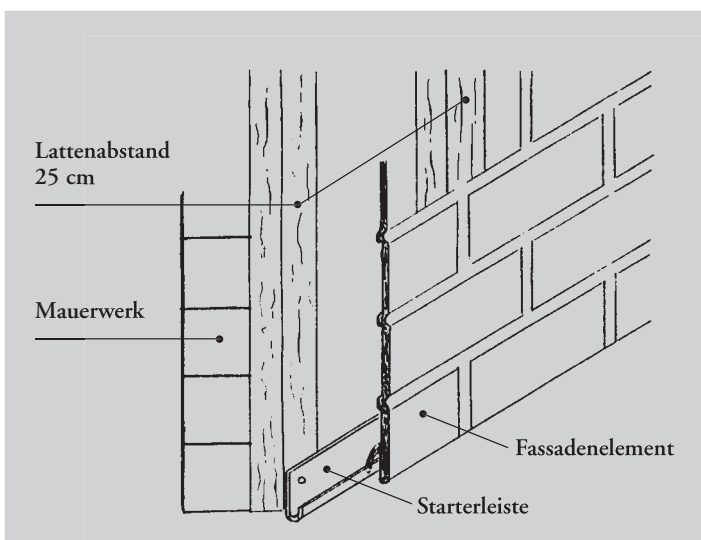
Aufbau ohne Isolierung
