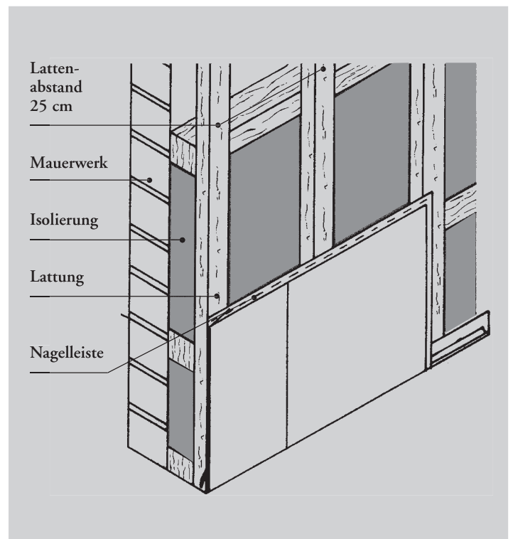
Aufbau mit Isolierung
