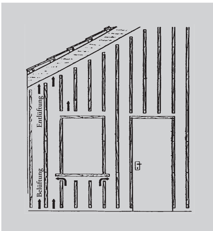
Be- und Entlüftung
