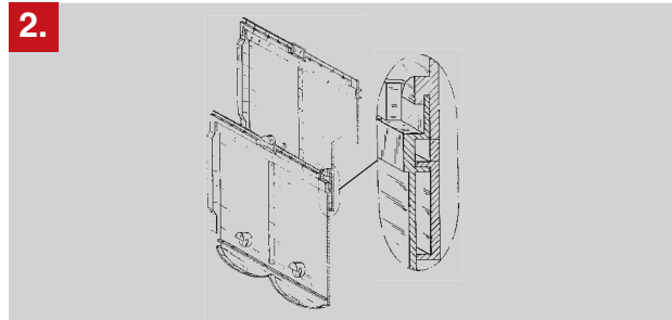
Rückansicht der Befestigung
