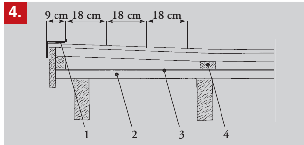
1 Ortgang angehoben, 2 Schalung, 3 Dachpappe, 4 Konterlatte
