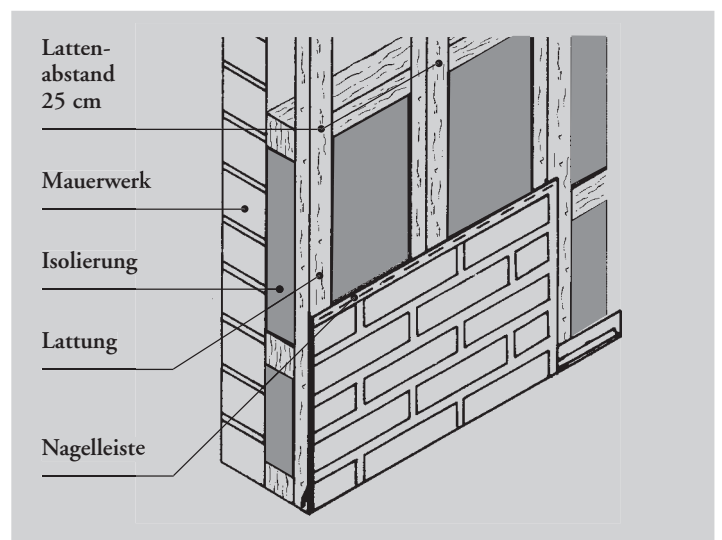
Aufbau mit Isolierung
