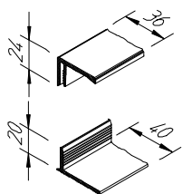
U-Profil 2-teilig
